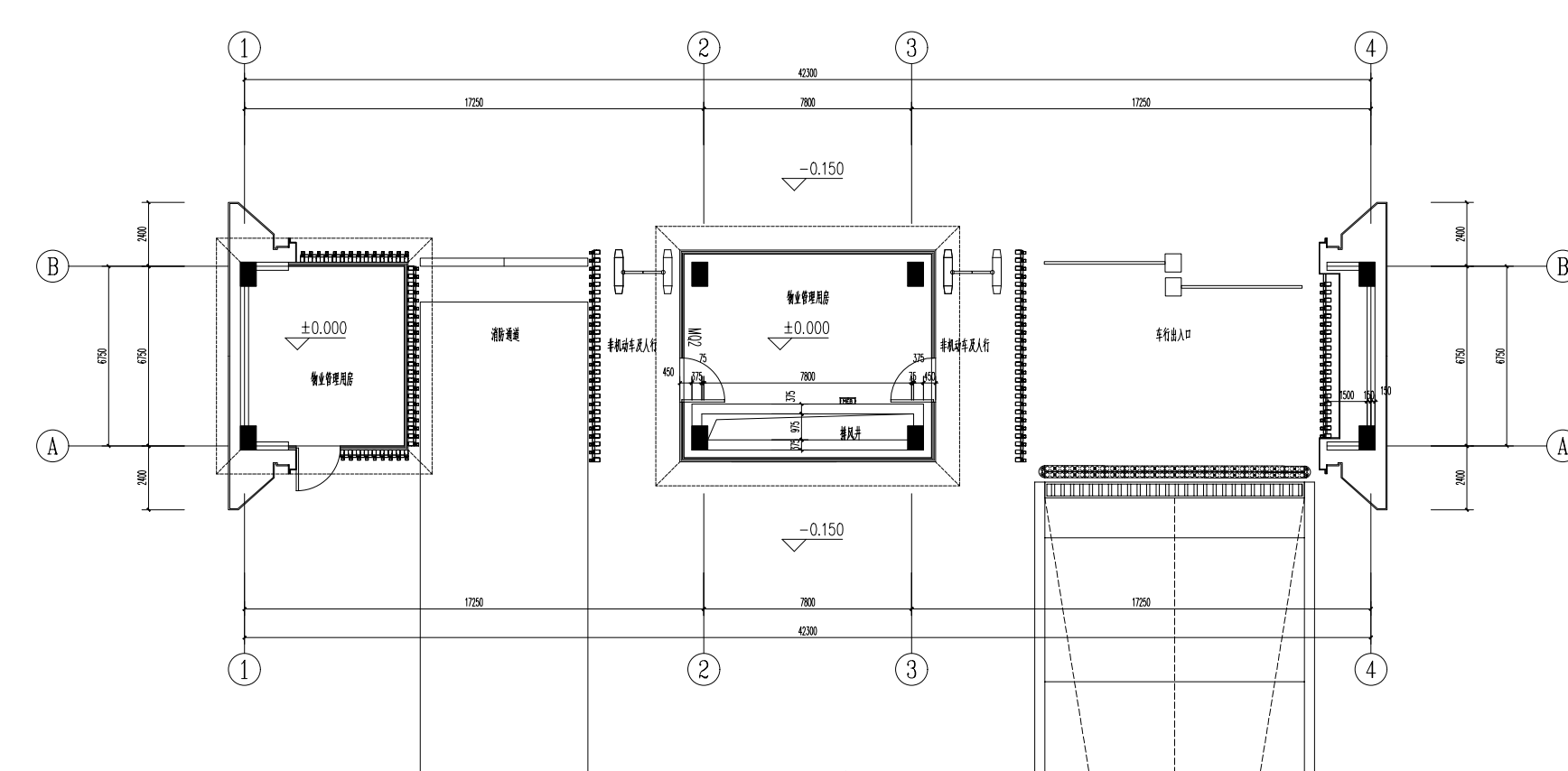
P5#楼一层平面图
